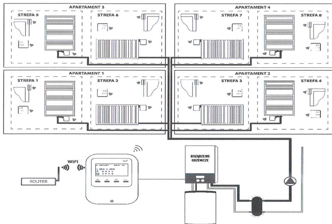
Rysunek. Schemat ideowy funkcjonowania systemu sterowania pracą układu c.o. w budynku
