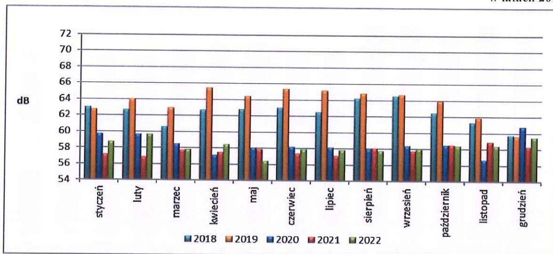
Zmiany długookresowego poziomu dźwięku L_{DWN} przy ul. Przy Kaszowniku w latach 2018-2022
