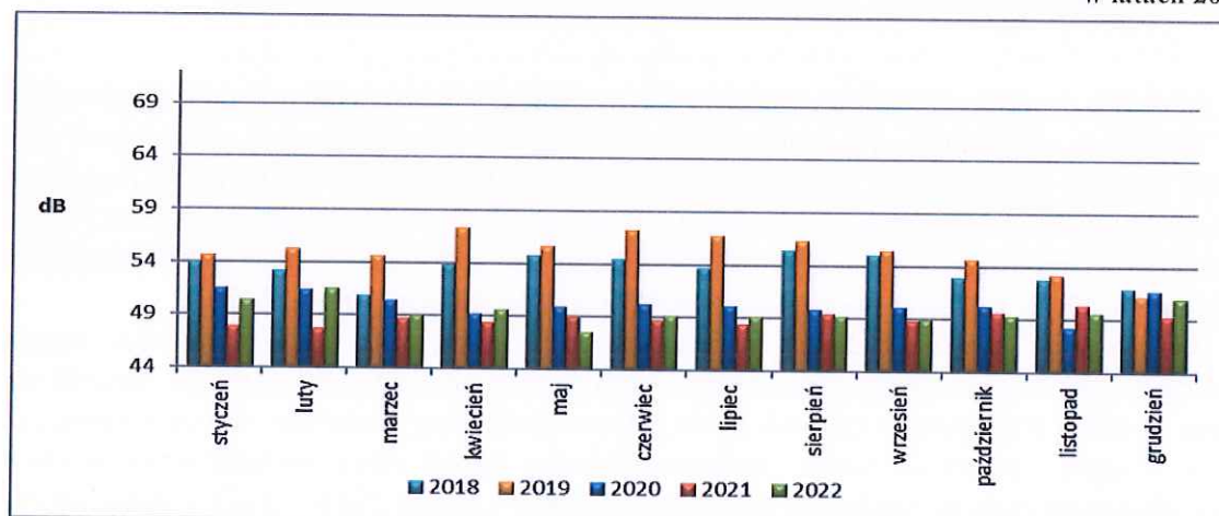
Zmiany długookresowego poziomu dźwięku L_N przy ul. Przy Kaszowniku w latach 2018-2022
