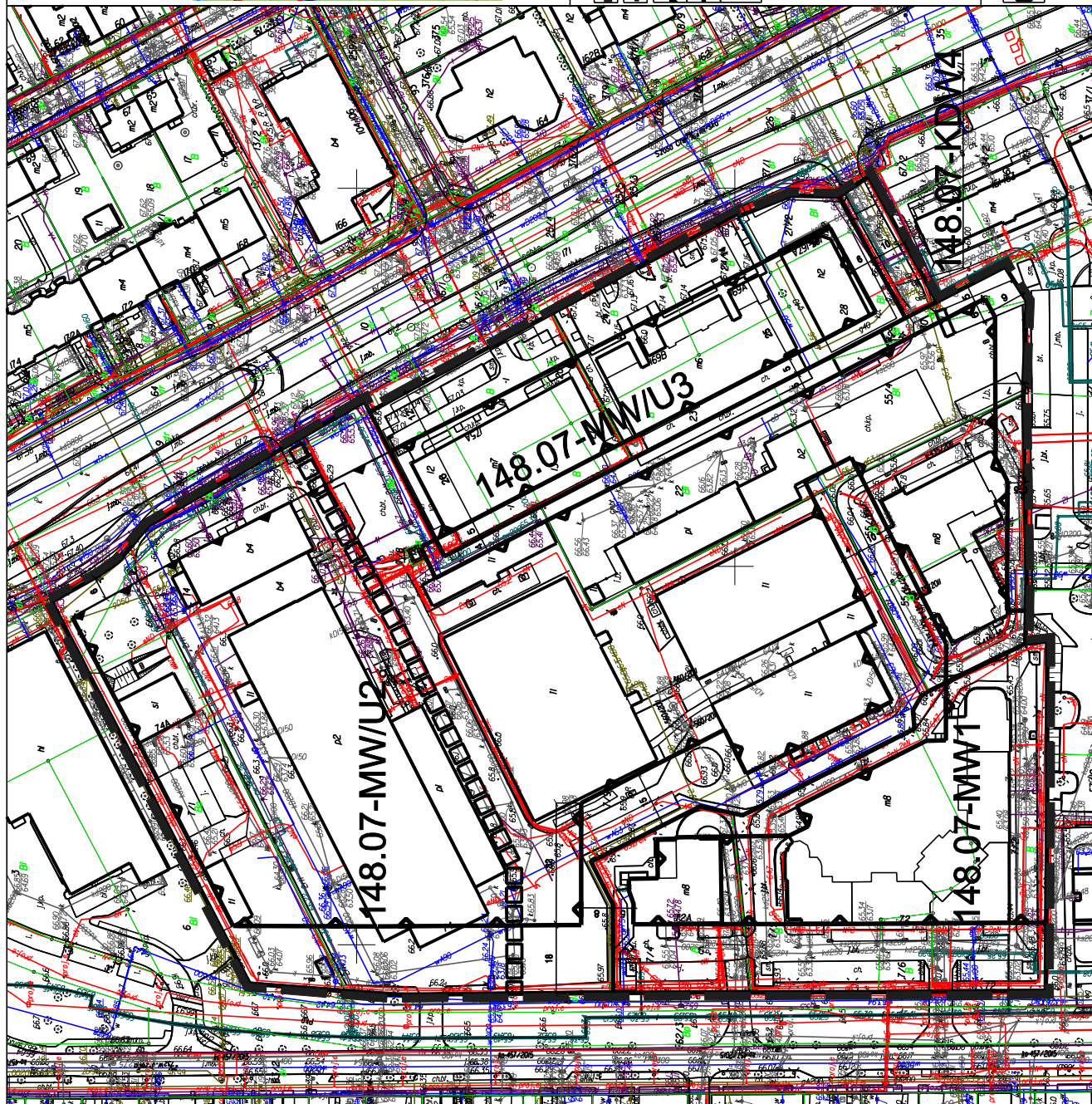
RYSUNEK PLANU SKAŁA 1:1000
